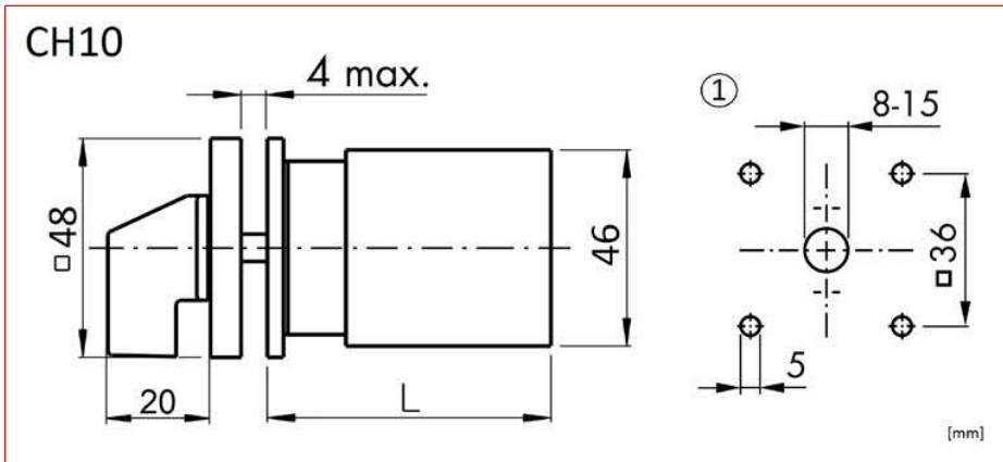
1) Bohrplan
