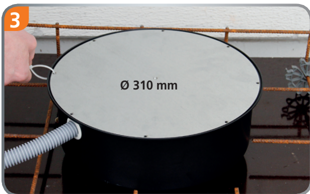
Rohre/Kabel einführen und stabile Blechplatte mit Kabelbinder befestigen.
