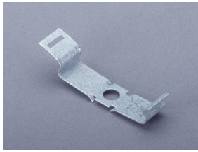
08 825 Schnappbefestigung für Tragschiene 35 x 7,5
