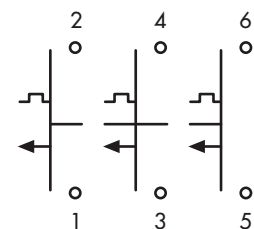
SCHALTBILD
