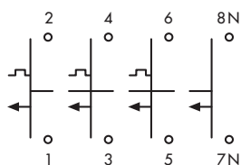
SCHALTBILD
