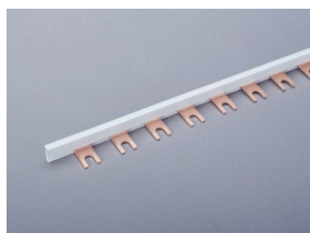
31 024 Kammschiene 1-polig, isoliert, Gabel 80 A, Teilung 27 mm, 1 m lang 16 mm 2
