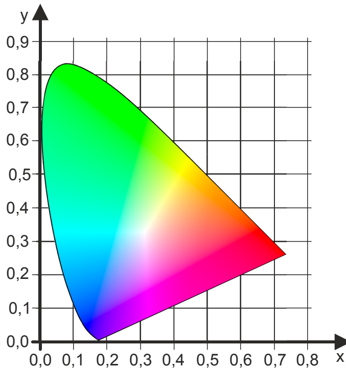
Abb. 9: Koordinatensystem des CIE-Normfarbraums
