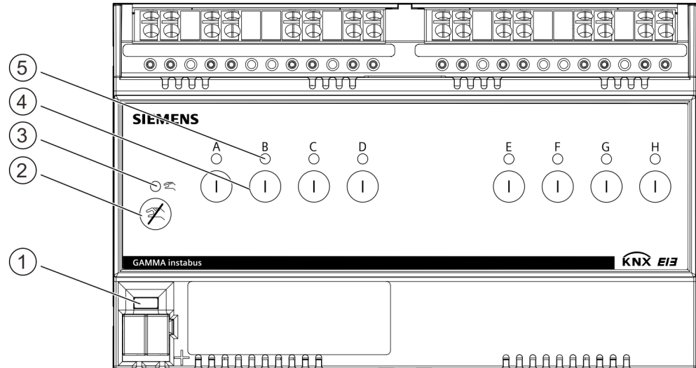
Abb. 1: Bedien- und Anzeigeelemente, Beispiel: Binäreingang 8 x potentialfrei
