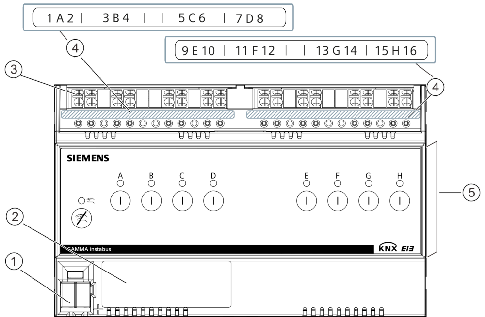
Abb. 2: Lage und Funktion der Anschlüsse und Beschriftung, Beispiel: Binäreingang 8 x potentialfrei
