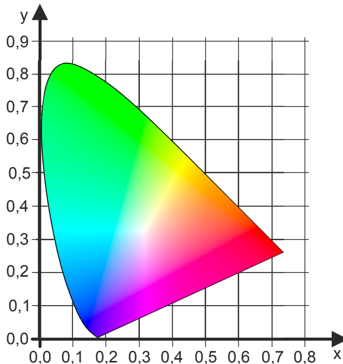
Abb. 12: Koordinatensystem des CIE-Normfarbraums
