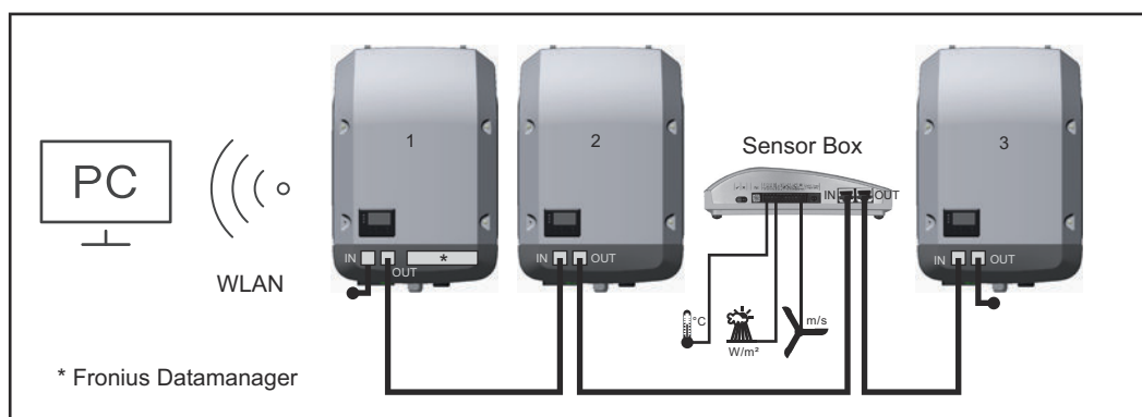
Datatenetwerk met 3 omvormers en een Fronius Sensor Box:
