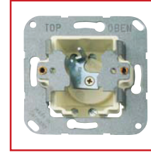
Schlüsseltaster-Einsatz
