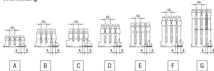
Seitenstanzung:
