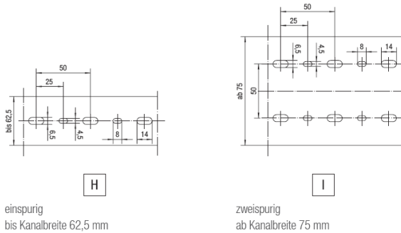
Bodenstanzung nach DIN 43659:
