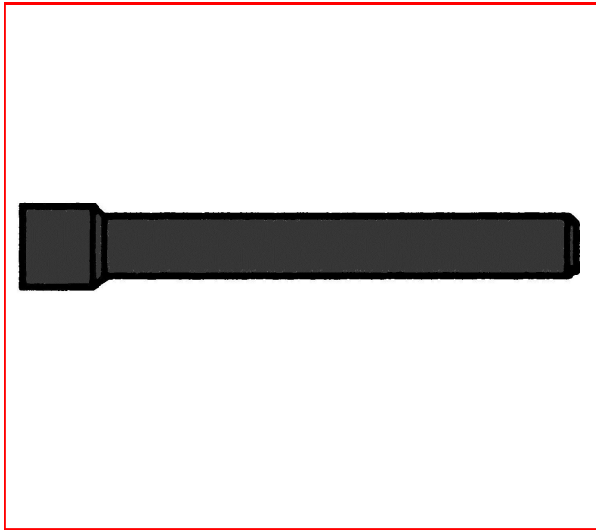
GTKSR
