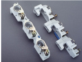
01 492 CUSTO® 60Classic D0-Reiter-Sicherungssockel, 27mm für Schiene 10 mm E 18 / 3P
