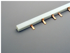
31 310 Kammschiene 3-polig, isoliert 80 A, Teilung 40 mm, 1 m lang 16 mm 2
