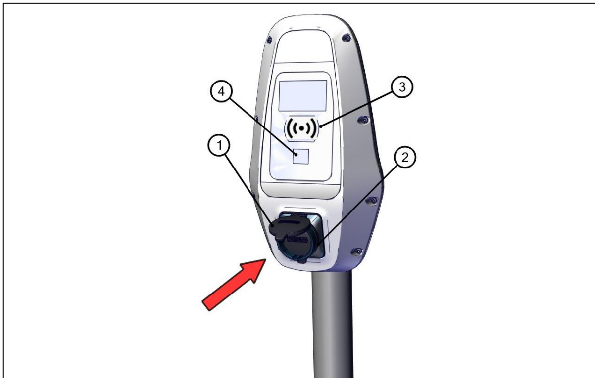
Bild 19 Ladebuchse
