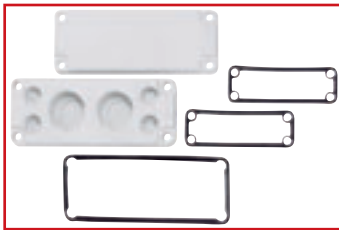
FLANSCH-GRUPPE
