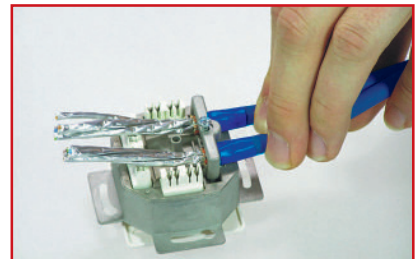
Den Bügel zur Befestigung der Kabel aufsetzen. / Put cable clip ready for fixing of cables.
