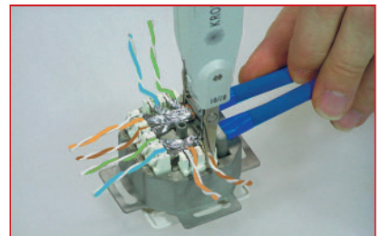
Die einzelnen Adern mit LSA Werkzeug (Art. Nr.: HKRONELSA) aufschalten. / Apply wires by use of LSA-Tool (Order Code: HKRONELSA). Cut off excess length.
