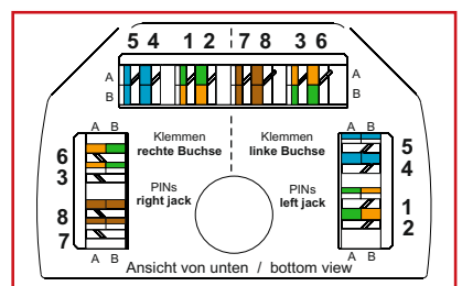
Verdrahtungsplan / Wiring diagram Nach / acc. EIA/TIA-568 A/B
