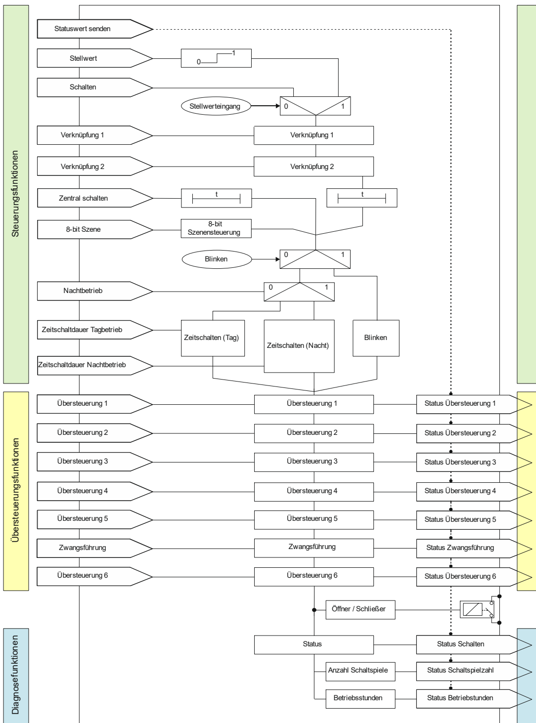
Schematischer Aufbau eines Schaltaktorkanals
