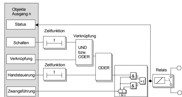
Bild 3: Blockschaltbild eines Ausgangs im Normalbetrieb
