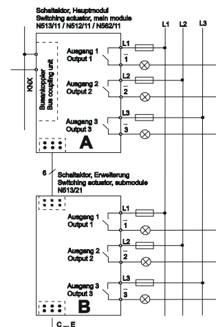
Bild 1: Schaltaktor-Hauptmodul und -Erweiterung
