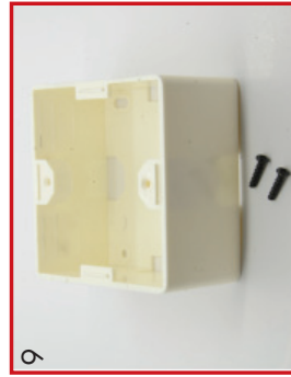
9 Aufputzrahmen HSEAP842WF und Schraubenset HSEDZBES / Wallmount frame HSEAP842WF and set of screws HSEDZBES
