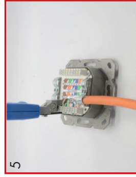
5 Adern mit LSA-Werkzeug HSKRONELSA aufschalten / Terminate the wires with LSA-tool HSKRONELSA
