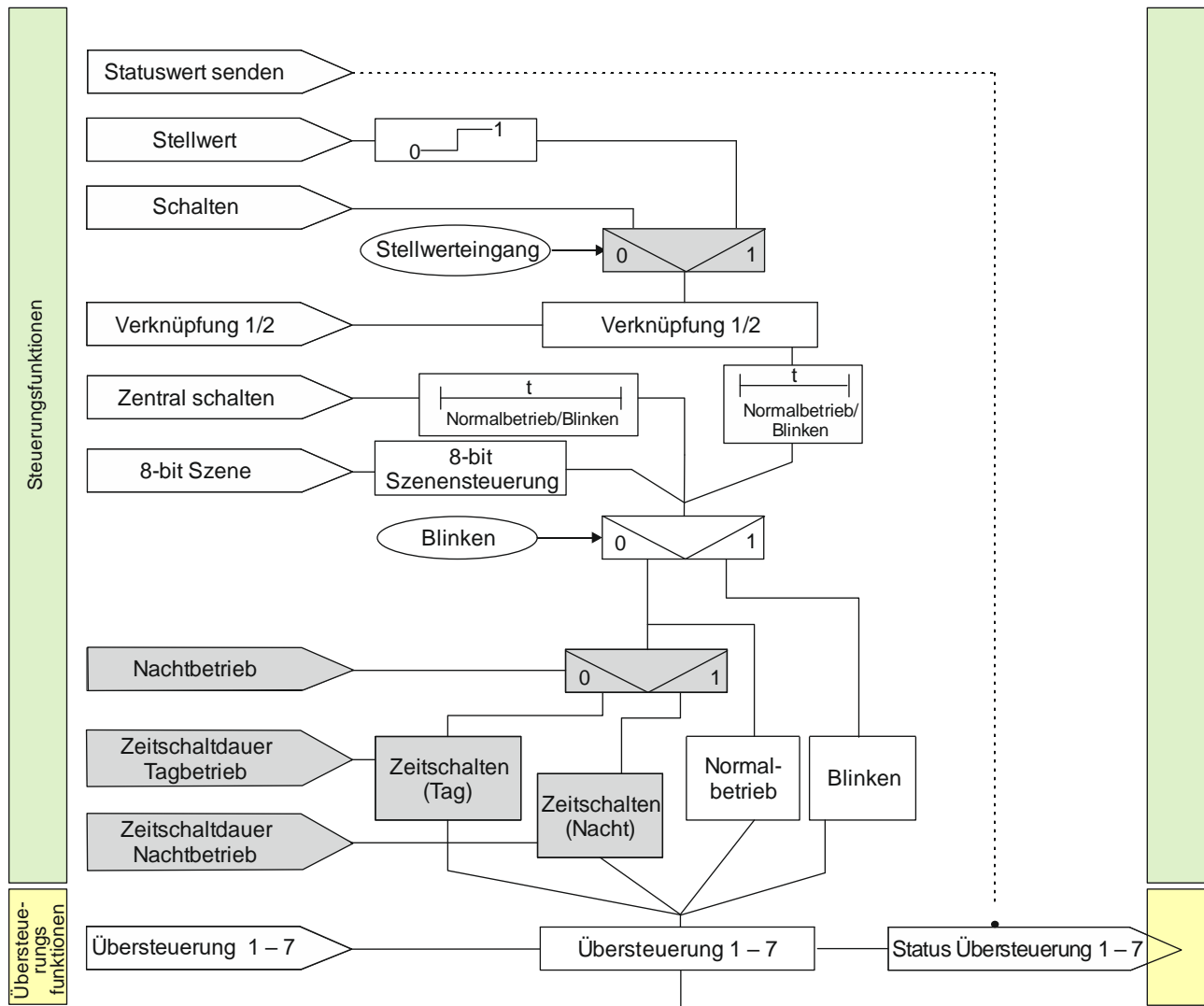
Abb. 4 Zeitschalterbetrieb
