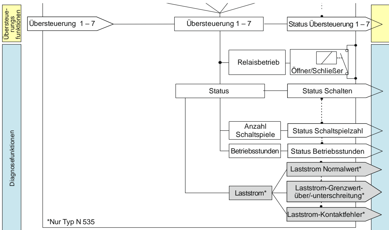
Abb. 25 Laststrom
