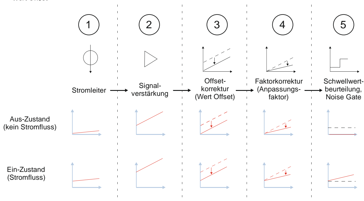
Abb. 20 Wirkung von Offset und Anpassungsfaktor bei der Strommesswerterfassung
