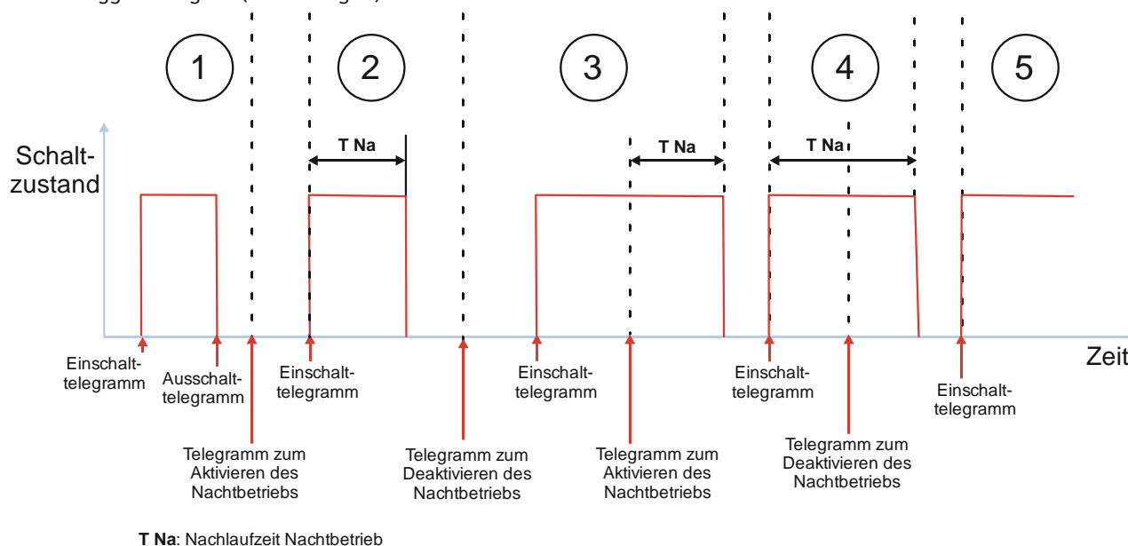
Abb. 36 Verhalten bei Aktivierung und Deaktivierung des Nachtbetriebs im Normalbetrieb
