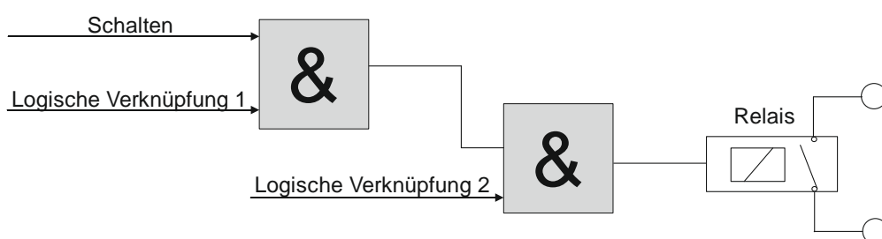
Abb. 6 Logische Verknüpfungen für den Kanal A
