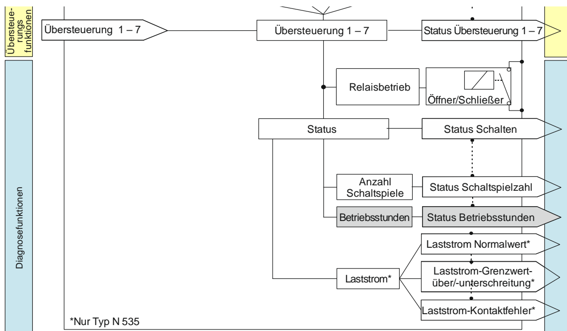
Abb. 28 Betriebsstundenzählung (Übersicht)
