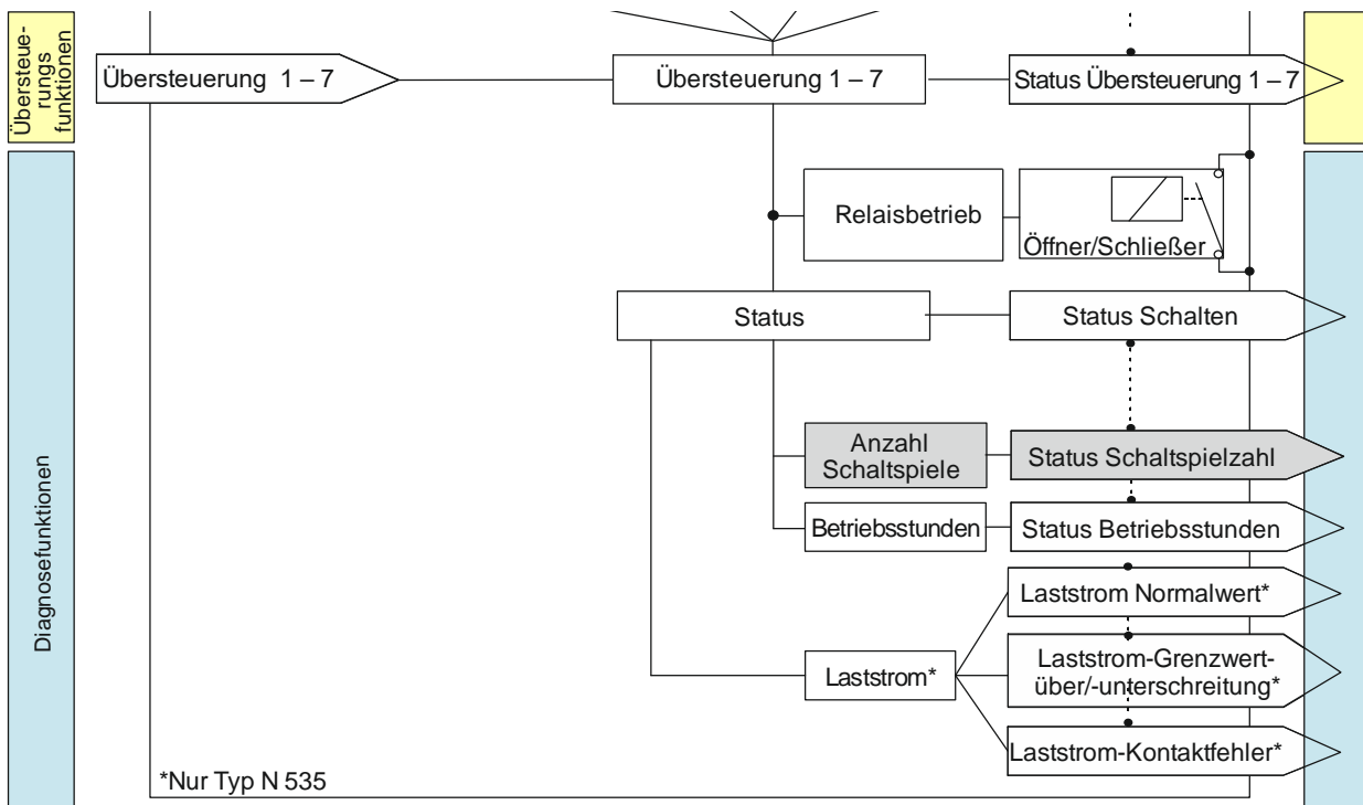
Abb. 26 Schaltspielzählung (Übersicht)
