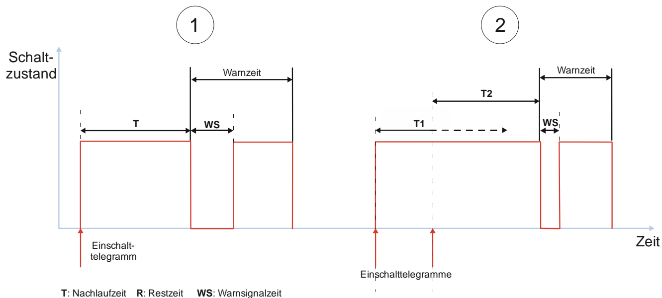
Abb. 34 Verhalten bei Zeitschalterbetrieb mit Einstellung „Warnen vor Ausschalten“ = „kurzes Aus-/Einschalten“ und „Nachtriggern möglich“ = „1“
