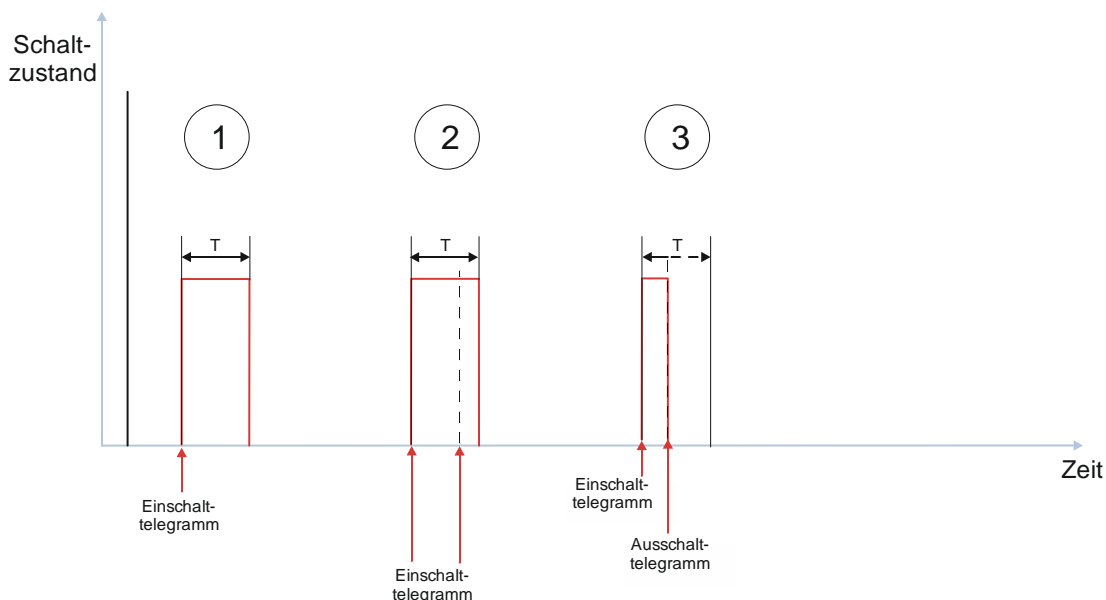
Abb. 30 Verhalten bei Zeitschalterbetrieb mit Einstellung „Nachtriggern = 0“
