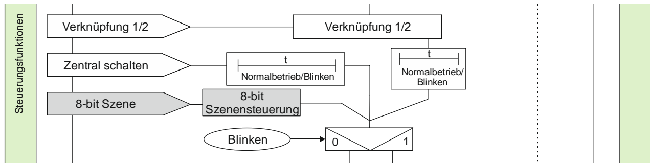
Abb. 10 8-bit Szenensteuerung
