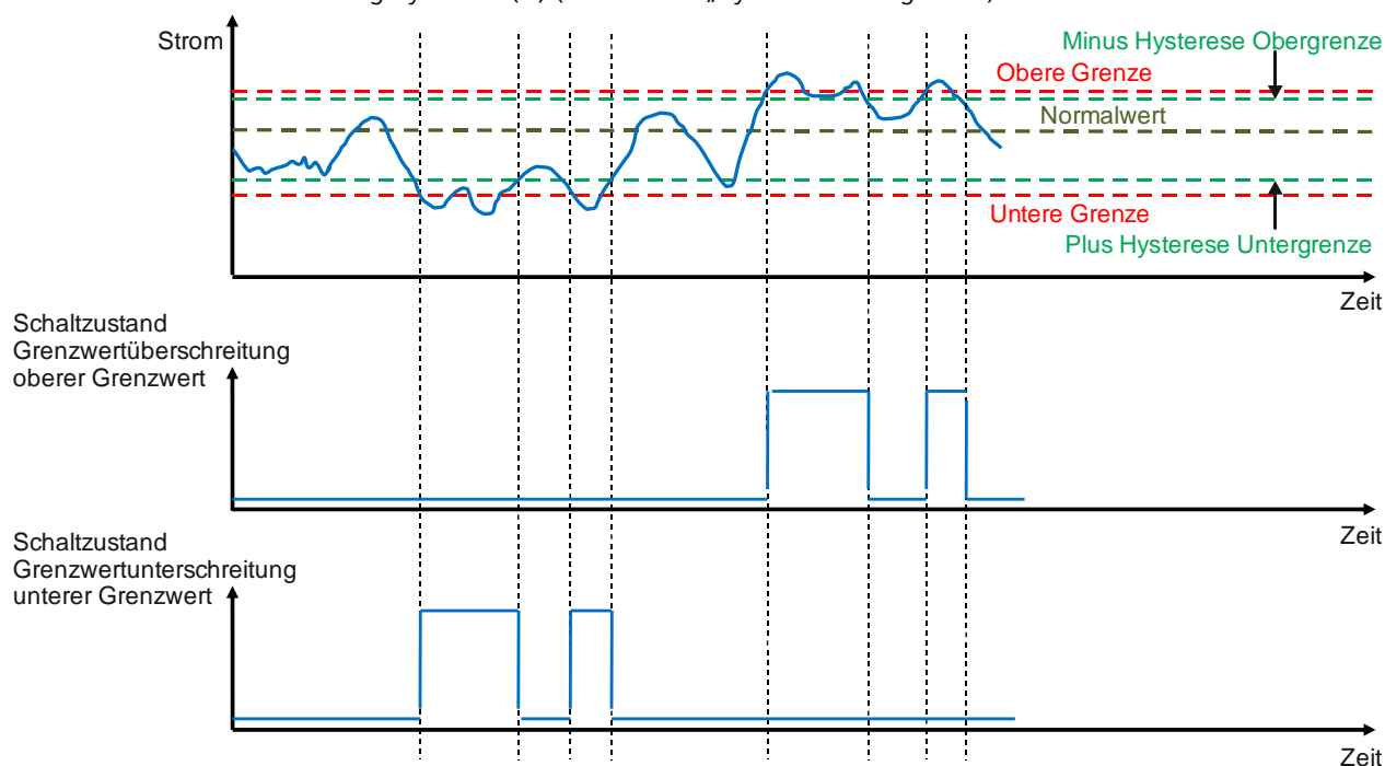
Abb. 21 Diagrammdarstellung Laststromüberwachung
