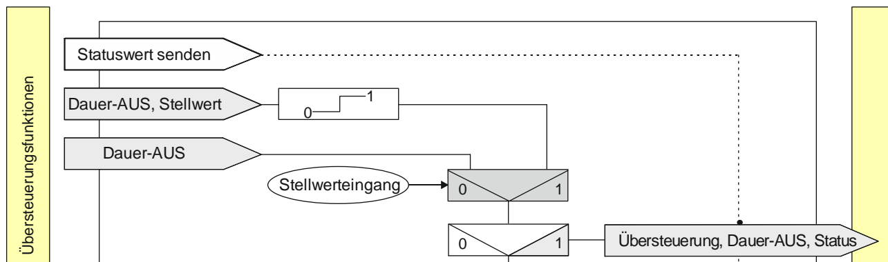
Abb. 14 Übersteuerung „Dauer-AUS“
