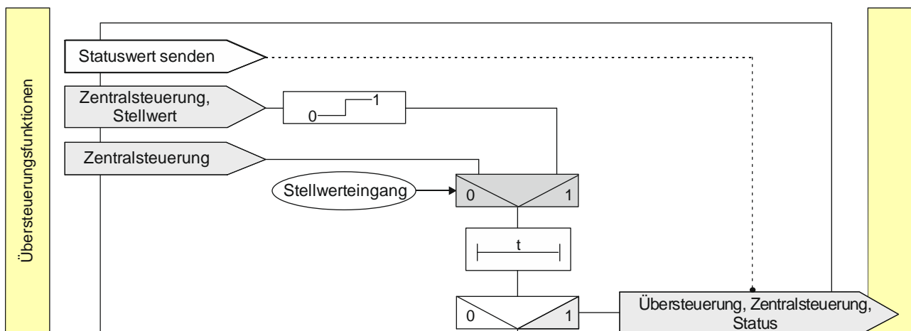
Abb. 16 Zentralübersteuerung
