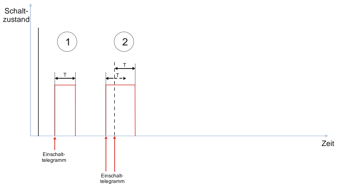
Abb. 31 Verhalten bei Zeitschalterbetrieb mit Einstellung „Nachtriggern = 1“
