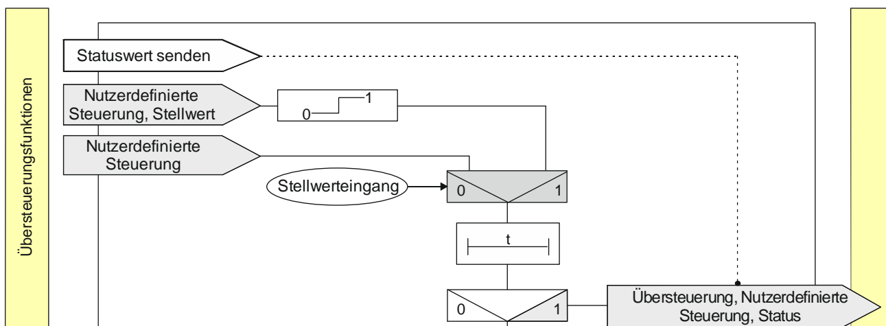
Abb. 17 Übersteuerung Nutzerdefinierte Steuerung
