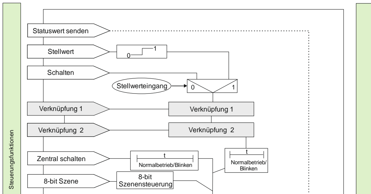
Abb. 7 Logische Verknüpfungen
