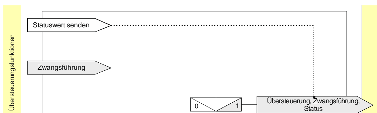
Abb. 18 Zwangsführung
