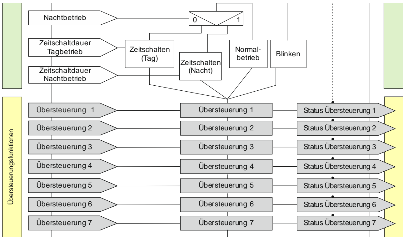
Abb. 12 Übersteuerungen
