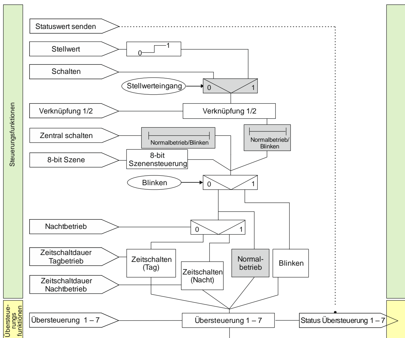
Abb. 3 Normalbetrieb
