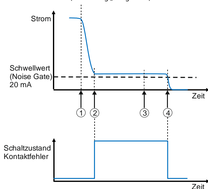
Abb. 24 Kontaktfehler
