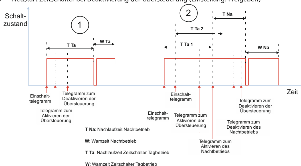
Abb. 41 Verhalten des Schaltaktors im Zeitschalterbetrieb mit Nachtbetrieb, parametrierter Übersteuerung (Zwangsführung) und Vorgabe zum Neustart des Zeitschalters bei Deaktivierung der Übersteuerung
