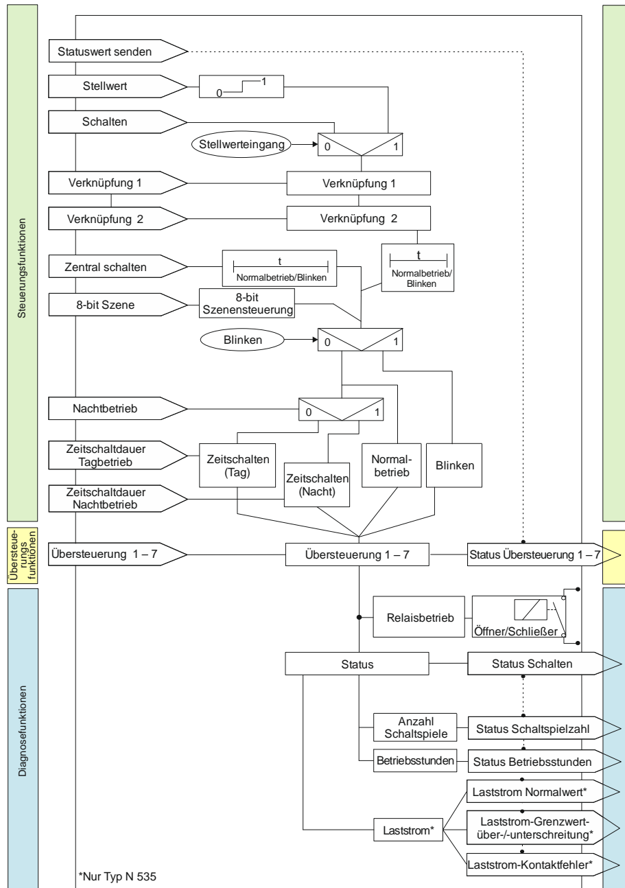
Abb. 1 Schematischer Aufbau eines Schaltaktorkanals (es werden nicht alle Kommunikationsobjekte dargestellt)
