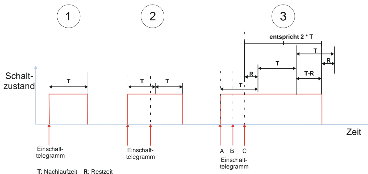
Abb. 32 Verhalten bei Zeitschalterbetrieb mit Einstellung „Nachtriggern möglich“ = „2“
