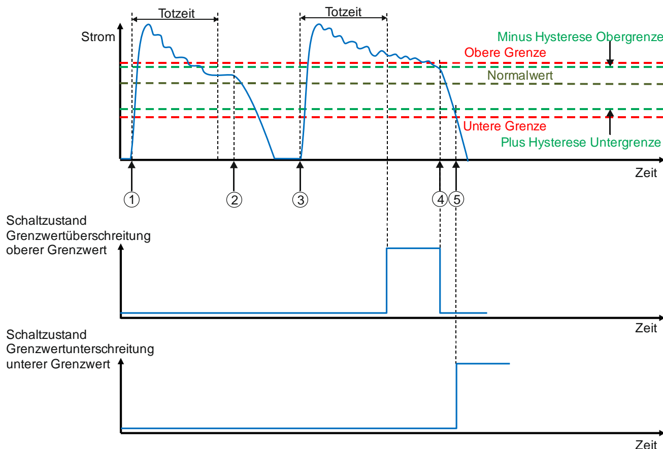
Abb. 23 Darstellung Grenzwertüberwachung mit Totzeit
