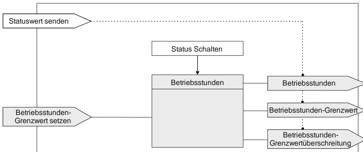
Abb. 29 Betriebsstundenzählung (Details)
