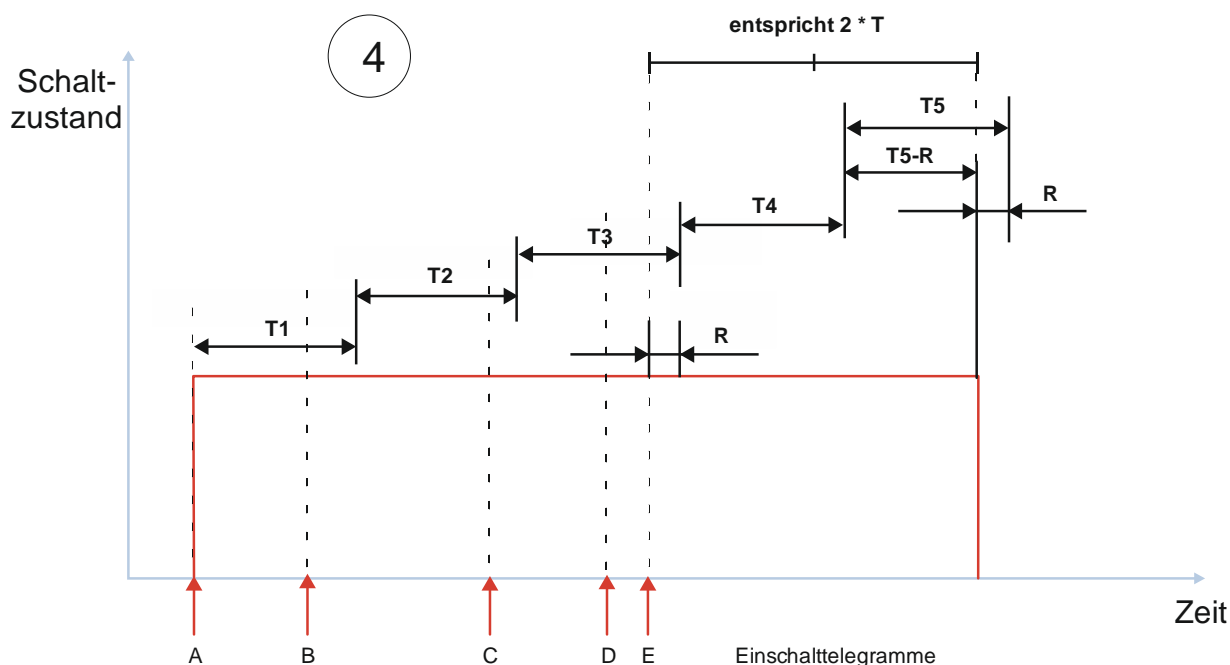
Abb. 33 Verhalten bei Zeitschalterbetrieb mit Einstellung „Nachtriggern möglich“ = „2“
