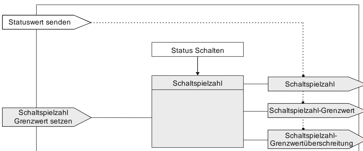
Abb. 27 Schaltspielzählung (Details)
