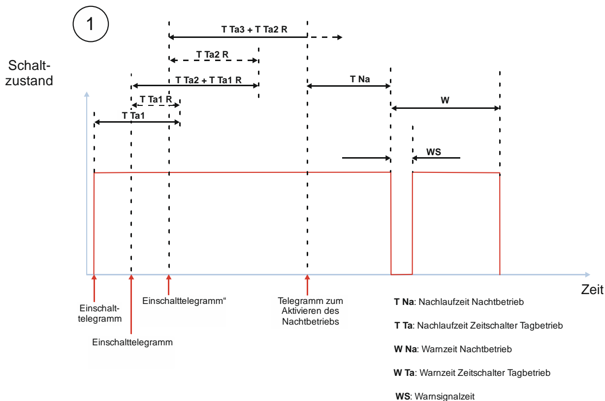
Abb. 37 Verhalten bei Aktivierung und Deaktivierung des Nachtbetriebs im Zeitschalterbetrieb
