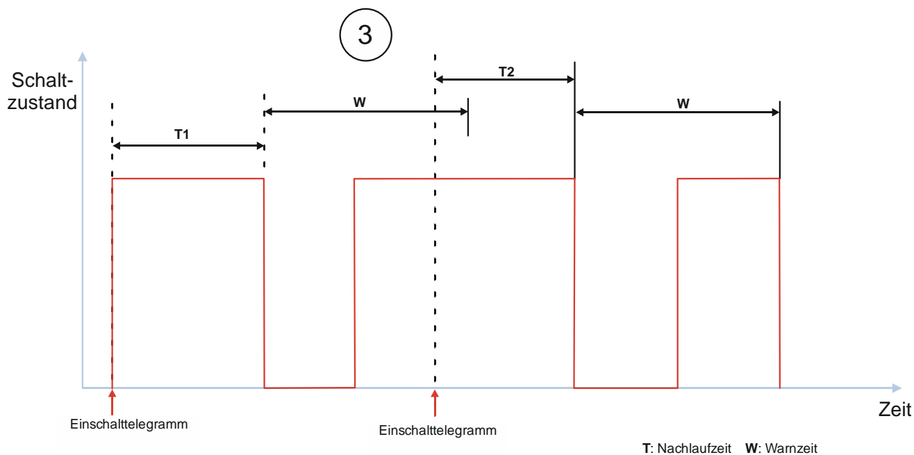
Abb. 35 Verhalten bei Zeitschalterbetrieb mit Einstellung „Warnen vor Ausschalten“ = „kurzes Aus-/Einschalten“ und „Nachtriggern möglich“ = „1“
