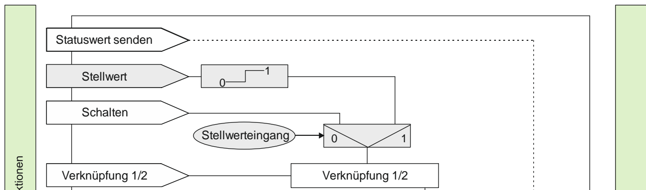
Abb. 8 Funktion Stellwerteingang
