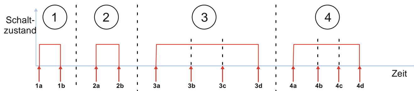
Abb. 39 Verhalten der Übersteuerungen des Kanals beim „Ein-/Ausschalten“ (Beispiel mit Übersteuerung „Hand EIN“)
