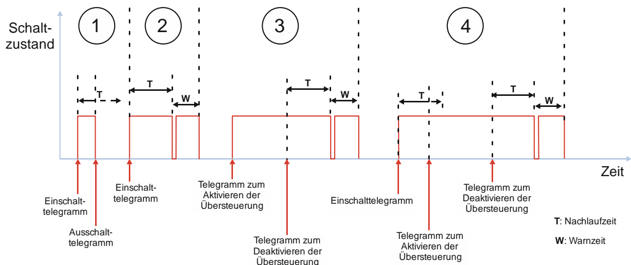
Abb. 40 Verhalten des Schaltaktors im Zeitschalterbetrieb bei parametrierter Übersteuerung (Zwangsführung) und Vorgabe zum Neustart des Zeitschalters bei Deaktivierung der Übersteuerung
