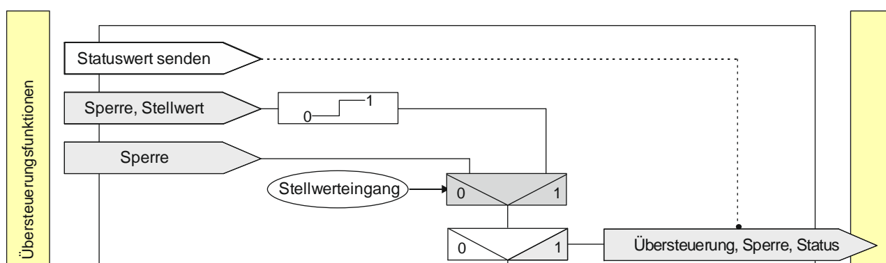
Abb. 15 Übersteuerung Sperre
