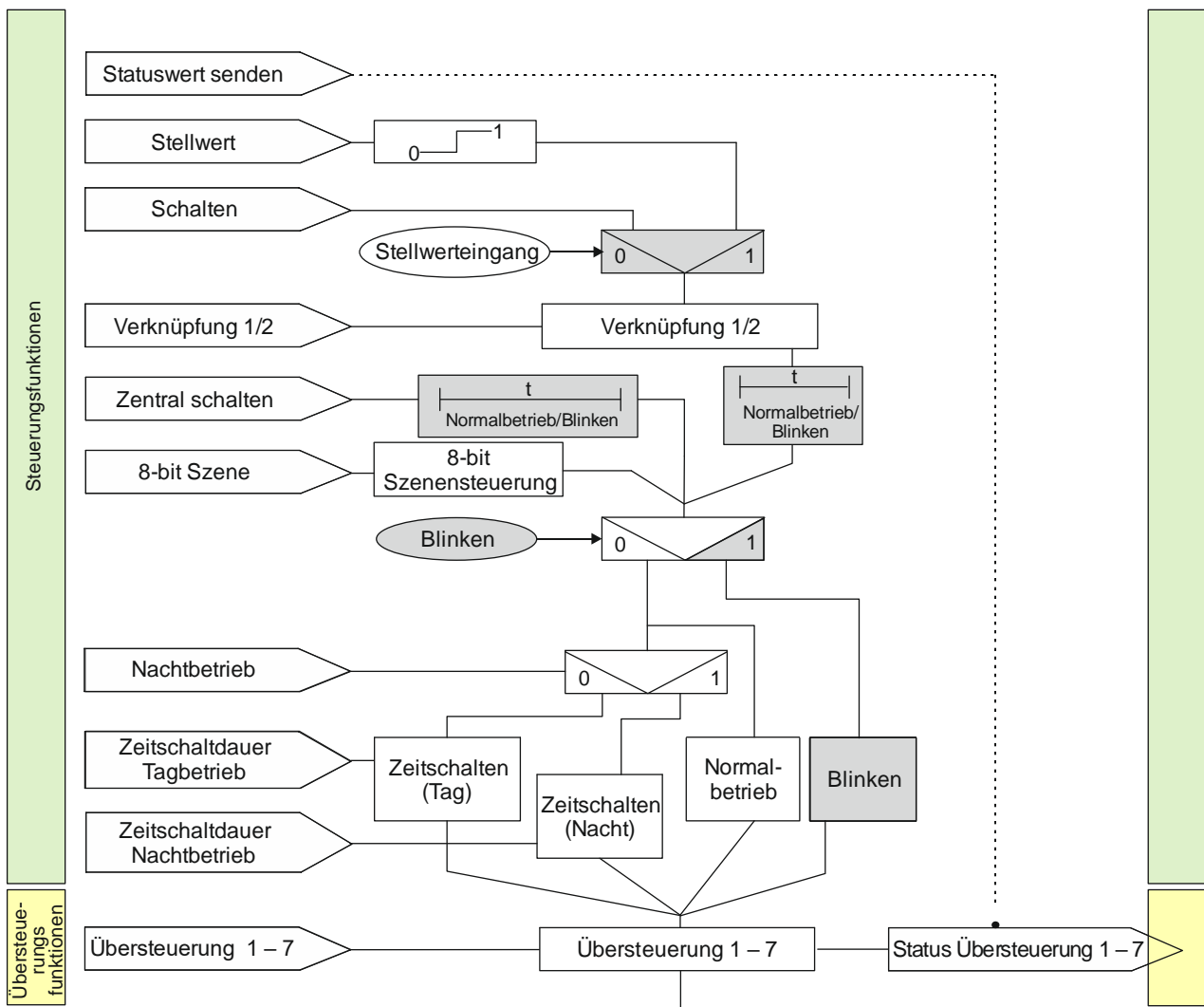
Abb. 5 Blinken
