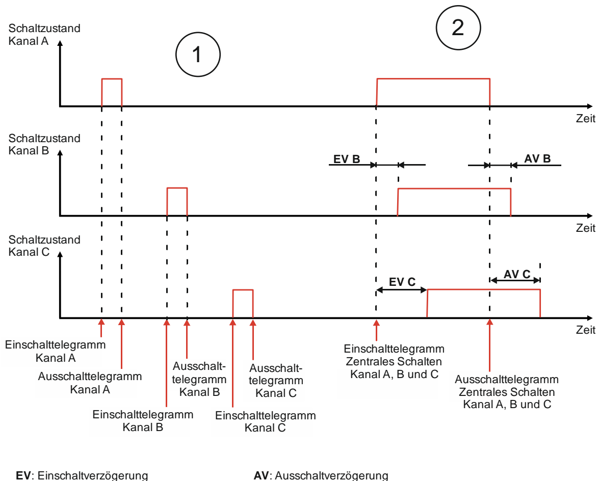
Abb. 42 Verhalten der Kanäle beim Schalten über das Kommunikationsobjekt „Zentrales Schalten“ mit Zeitverzögerung
