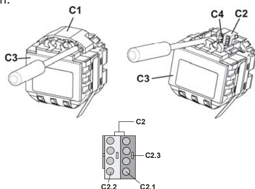
Bild 4: Busklemme abziehen / aufstecken
