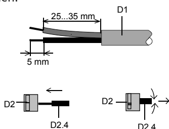
Bild 5: Anschließen / Abklemmen der Busleitung
